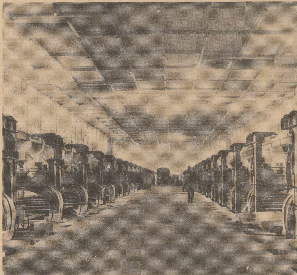
În această secție de electroliță de la Uzina de aluminiu Slatina, alumina expedită de Combinatul de la Oradea va fi transformată în curind în prodigiousul metal al.
