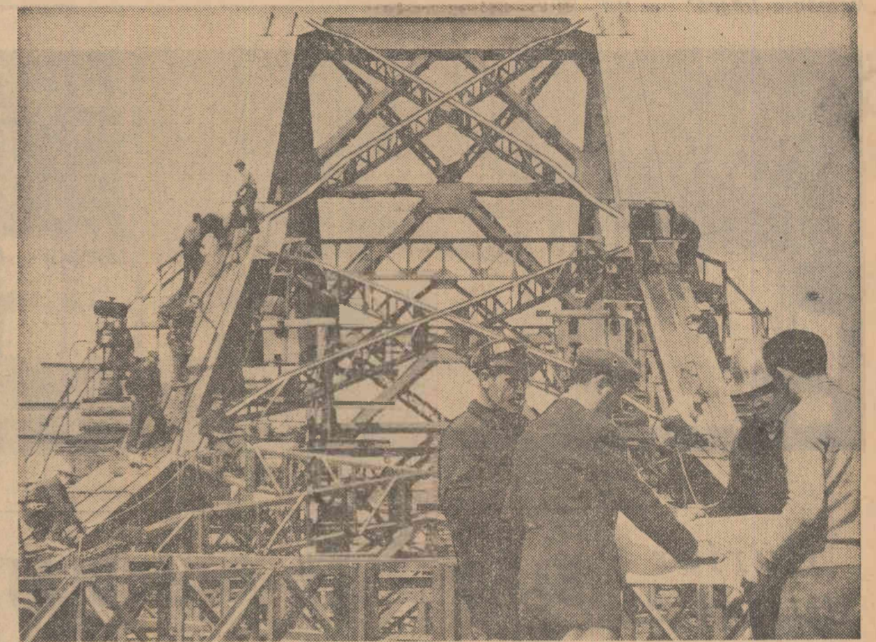
Lucrările de consolidare a podului de peste Borcea se află în faza finală. Ingerii Dumitru Stănescu și Mihale Dincu de la sanțierul de montaje din cadrul Direcției generale de construcții a Ministerului Transporturilor și Telecomunicațiilor, urmăresc împreună cu maistrul Voicu Borcan și brigadierul Ion Chelmeș aplicarea procesului tehnologic pentru consolidarea tălpii superioare a podului.
