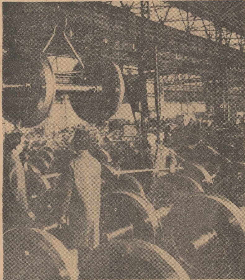
Secția osil montate tip C.F.R. de la uzinele „Progresul” din Brăila este frunțată pe întreprindere, depășindu-și în mod regulat sarcinile de plan și dând produse de bună calitate. În clișeu: Aspect din secție
