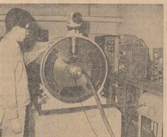
Aparat de fotografiat cu viteză foarte mare, capabil să fotografie instantanee pentru explozii, descărcări electrice, fuziuni nucleare. Acest aparat, care a fost construit în Japonia, are timp de expunere 1/500 000 din secundă și o viteză de fotografiere continuă între 200 și 600 imagini pe secundă. Camera, cu un sistem de lentile F8, are un diametru de 77 cm.
