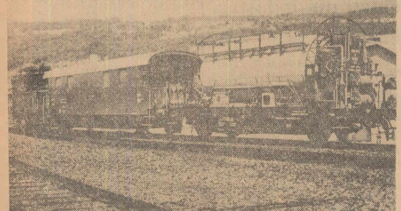
Un tren special de salvare este întrebuințat în Elveția în acțiunea de stingere a incendiilor izbucnite în tuneluri. Trenul special este compus dintr-o locomotivă, un vagon pentru transportarea echipelor de salvare în tunel și pentru transportul a maximum 50 de persoane salvate și un vagon special de transportat extincătoare chimice și oxigen
