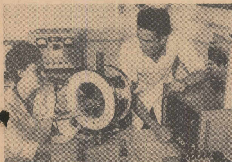
Sarcinile principale ale Institutului de metrologie constau în transmiterea unităților de măsură, omologarea aparatului de măsură, precum și în cercetări privind îmbunătățirea și mărirea preciziei măsurărilor. În clădire: Aspect din activitatea laboratorului de magnetometrie
