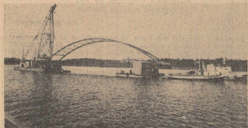
Construcția întregă a unui pod, cîntărînd 240 de tone, a fost, recent, transportată pe apă spre locul ei de amplasare din arhipelagul Stockholm. Acesta constituie primul transport al unui pod care a fost făcut vreodată pe apă în Suedia. Iată o imagine din timpul transportului pe apă al podului. Macarura plutitoare „Lodbroke” are pe puntea sa un capăt al podului, în timp ce cel de-al doilea capăt se află pe bordul unui bac, iar tracțiunea este executată de două motonave
