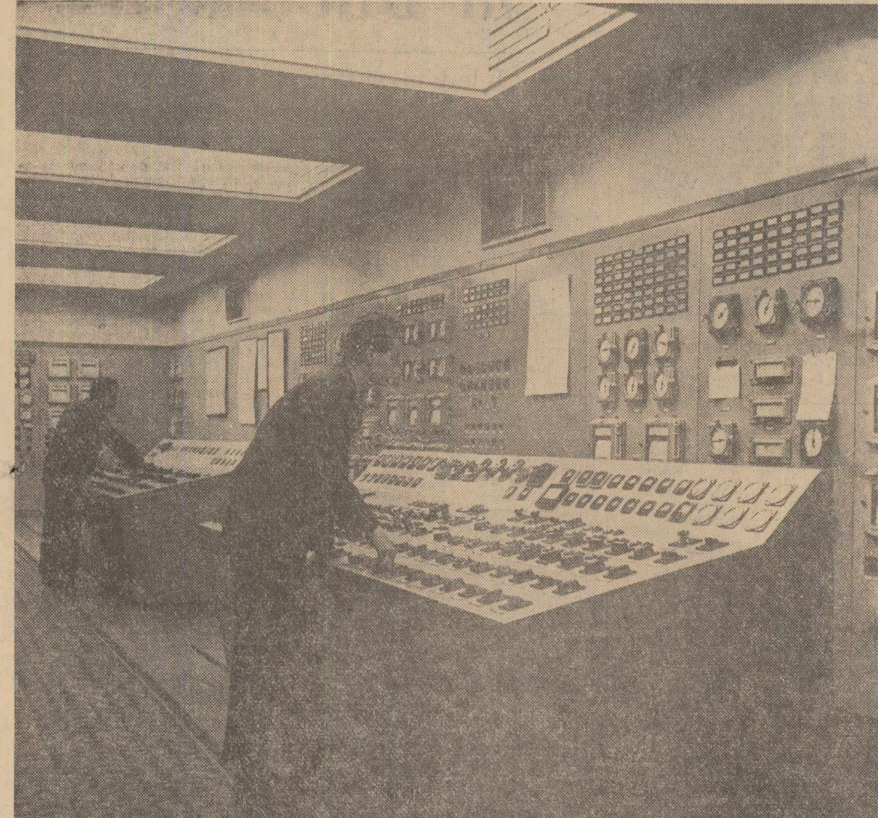
În București sînt în construcție o serie de obiective energetice al căror scop este îmbunătățirea alimentării cu energie electrică și termică a capitalei, extinderea termoficării urbane și industriale etc... La centrala electrică de termoficare Grozăvești, prin punerea în funcțiune a unui grup de 50 MW și a stației noi de 110 Kv, cu instalațiile lor auxiliare, capacitatea ei de producție a crescut cu 60 la sută. În prezent, centrala Grozăvești se execută lucrări de extindere cu încă un grup de 50 MW. În clișeu: aspect din camera de comandă termică a grupului de 50 MW. Foto: AGERPRES
