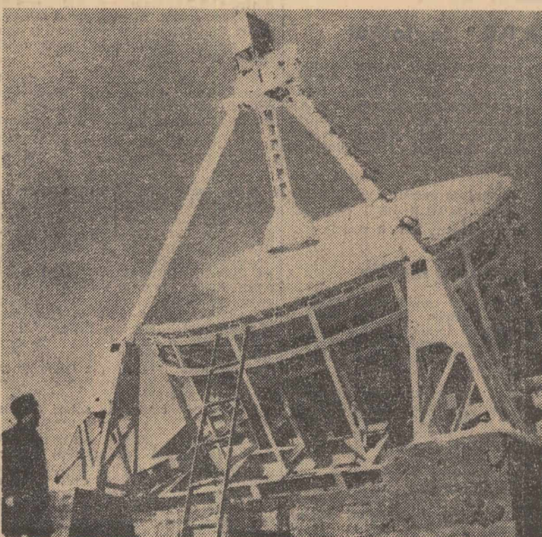
Instalarea de radiofizică și electronică la Academia de Științe a R.S.S. Armene a întocmit proiectul uneia din cele mai mari antene din lume, cu două oglinzi. Pe pînălul muntelui Aragat, nu departe de Observatorul astrofizic Biurocan, s-a terminat construcția modelului acestei antene.
