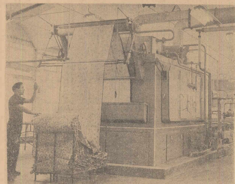
În sectorul de finisaj al întreprinderii textile „Dacia” din Capitală a fost dată recent în funcțiune o nouă instalație: cea de-a doua mașină specială pentru imprimat cu șablon pe pînă la 12 culori.
