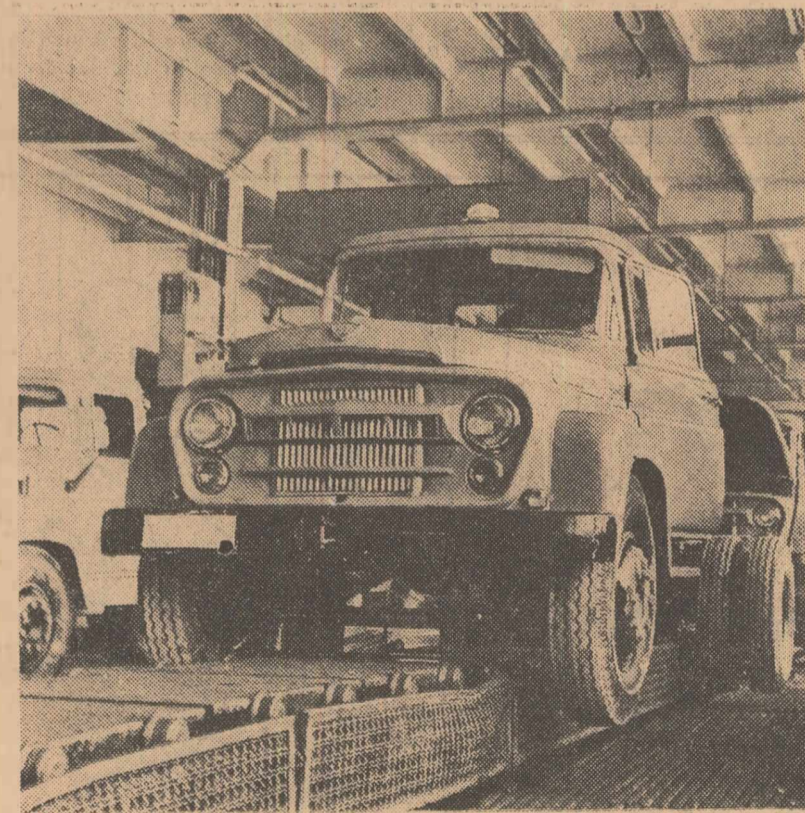
Autocamioane „Buick” de 5 tone, fabricate la uzinele „Steagul Roșu”, la coborîrea de pe convertorul de montaj general.
