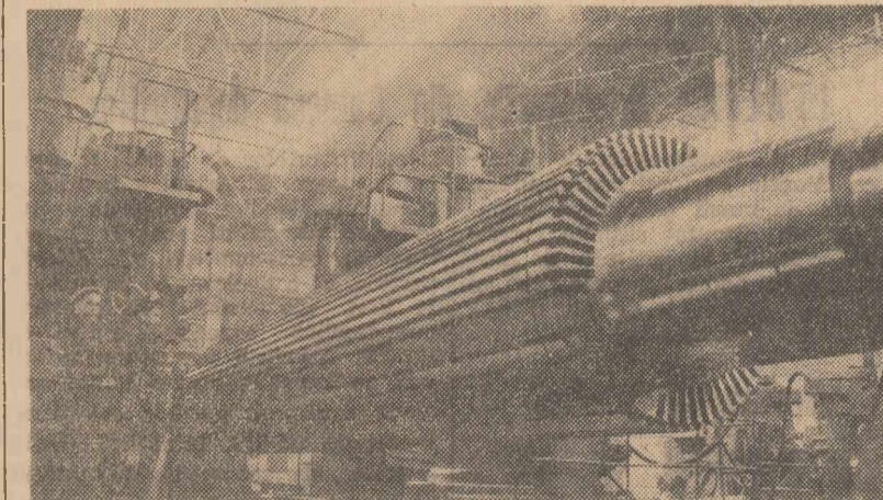
Realizarea unui turbogenerator cu o capacitate de 500 000 kw, unul din cele mai mari din lume, la Uzina electrotehnică „V. I. Lenin” din Harkov. În fotografie: prelucrarea rotorului turbogeneratorului la mașina de frezat
