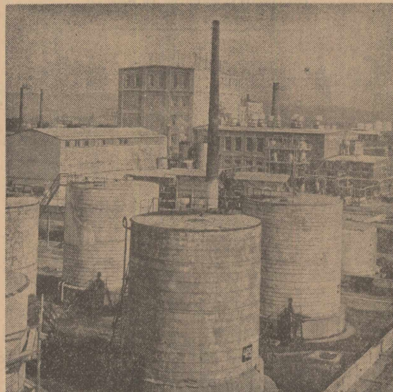
Vedere a instalației de contactare a uteiurilor din cadrul Rafinării Teleajen
