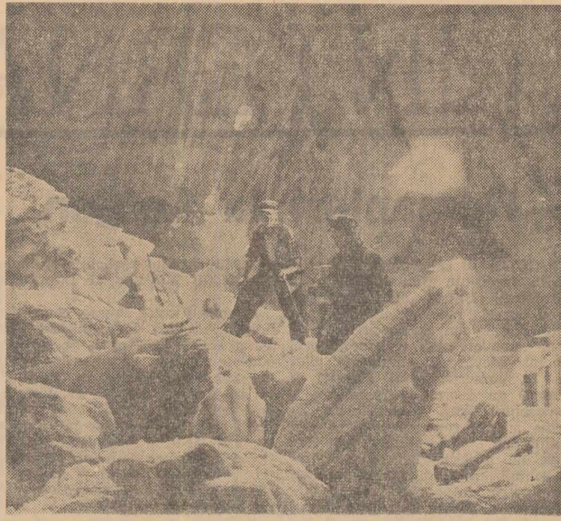
În saline, mecanizarea operațiilor de tăiere și de transport contribuie la creșterea productivității muncii. În cliseu: Stîncoile de sare din camerele de exploatare ale salinei Sălciu-Prahova sunt perforate pentru a fi încărcate în vagoane
