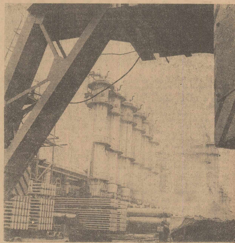
Coloanele de spălare a gazelor din cadrul fabricii de amoniac a Combinatului chimic Craiova
