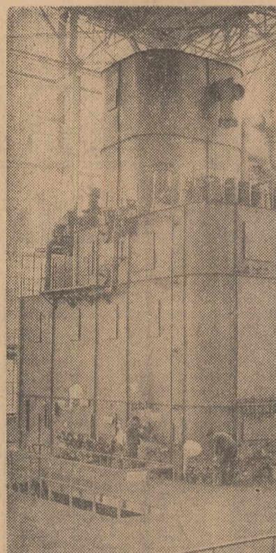
Pe șantierul Combinatului chimio Craiova, constructorii desfășoară din plin bătaia pentru a da în producție înainte de termen obiectivele prevăzute. De acum, au intrat parțial în funcțiune fabricile de amoniac și de oxigen. În cliseu: Blocul de separare a aerului din cadrul fabricii de oxigen
