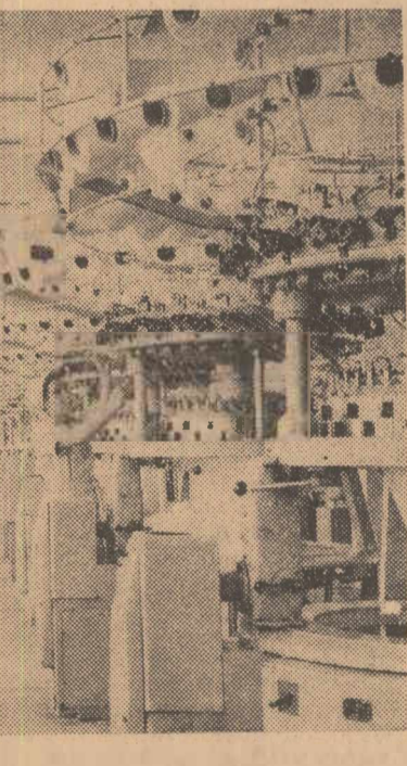
Uzinele textile „Moldova” din Iași produc o gamă variată de tricotate. În cliseu: Vedere din sala mașinilor de tricolat.
