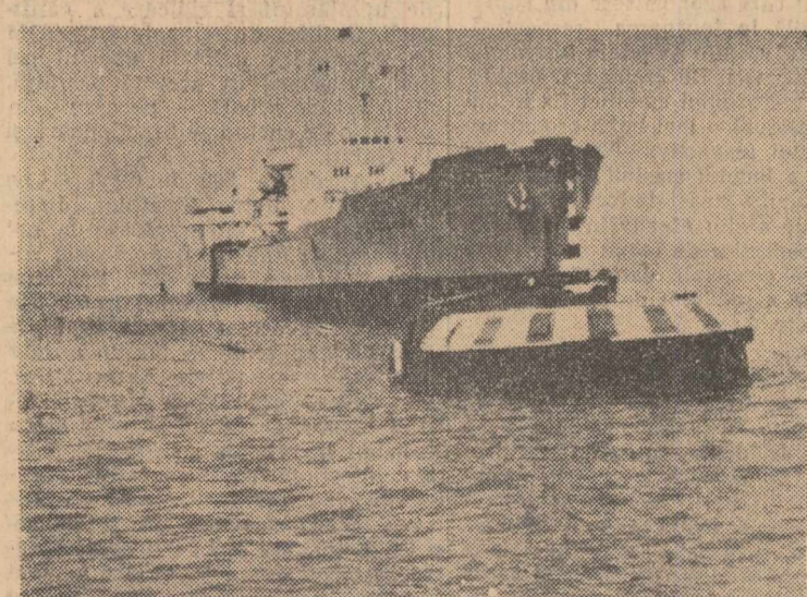
Geamandura „Imodco Terminal” construită în Suedia, cu ajutorul căreia pot fi descărcate tancurile petroliere direct din larg, fără ca ele să fie acostate la țărm. Încărcătura fluidă a unui tanc poate fi transportată în mod rapid prin conductele și tuburile prin care geamandura este în legătură cu țărmul
