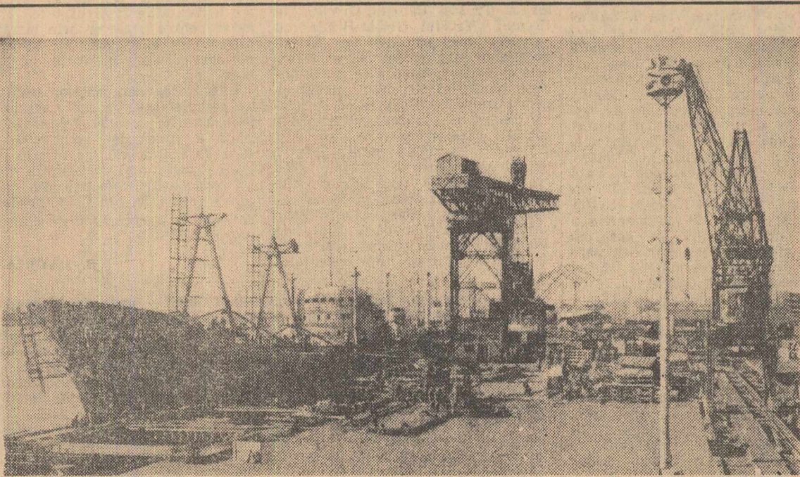
La cheiul de armare de la Șantierul naval Galați se montează instalațiile de încărcare-descărcare la un nou cargon de 4500 tone Foto: AGERPRES
