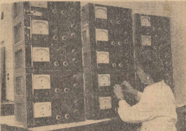
Institutul de Fizică Atomică. În clișeu: Redresori de înaltă tensiune pentru alimentarea fotomultiplicatorilor aflați pe bancul de probă
