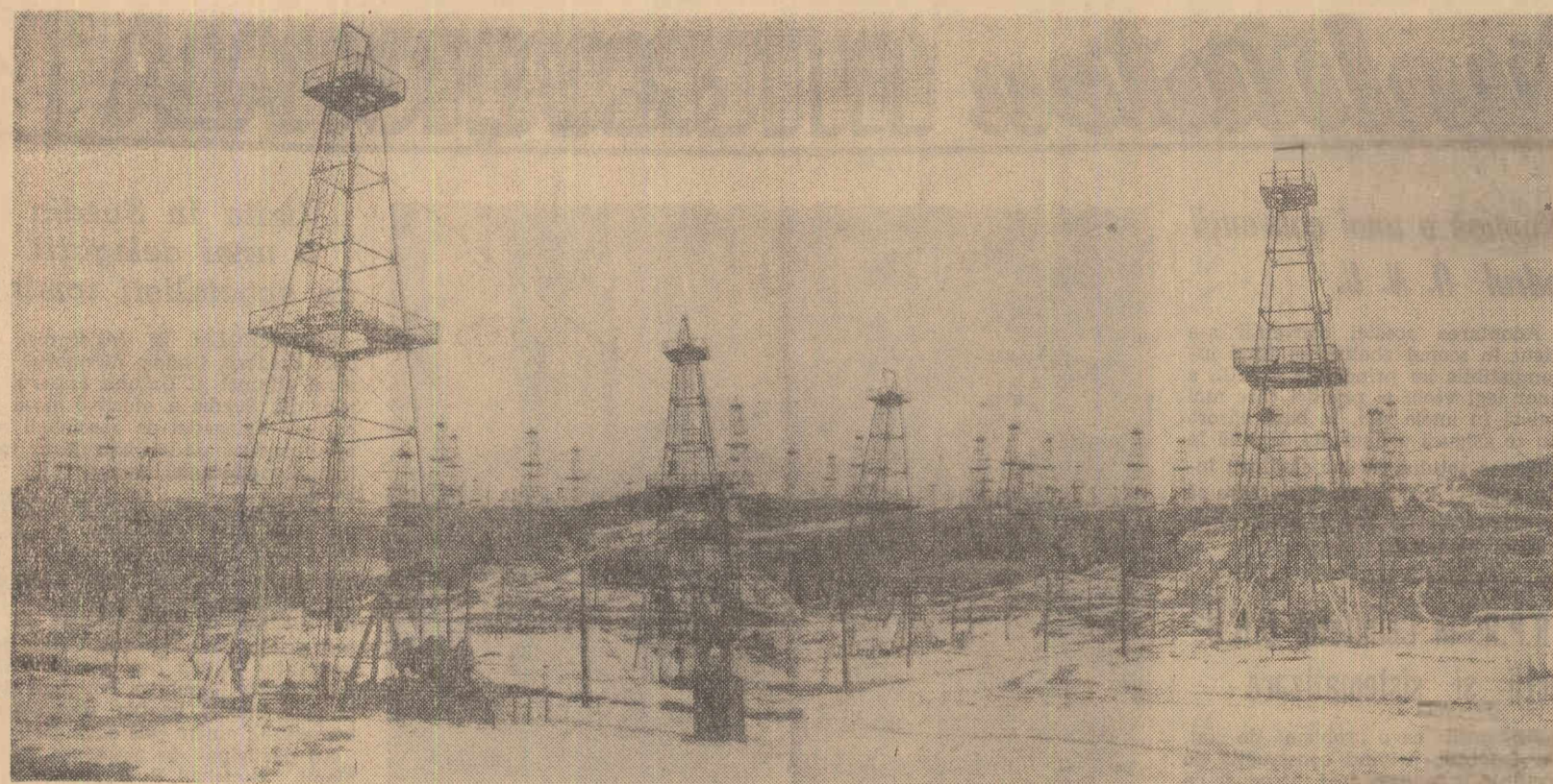
Cimp de sonde în schela de extracție Țicleni, regiunea Oltenia.
