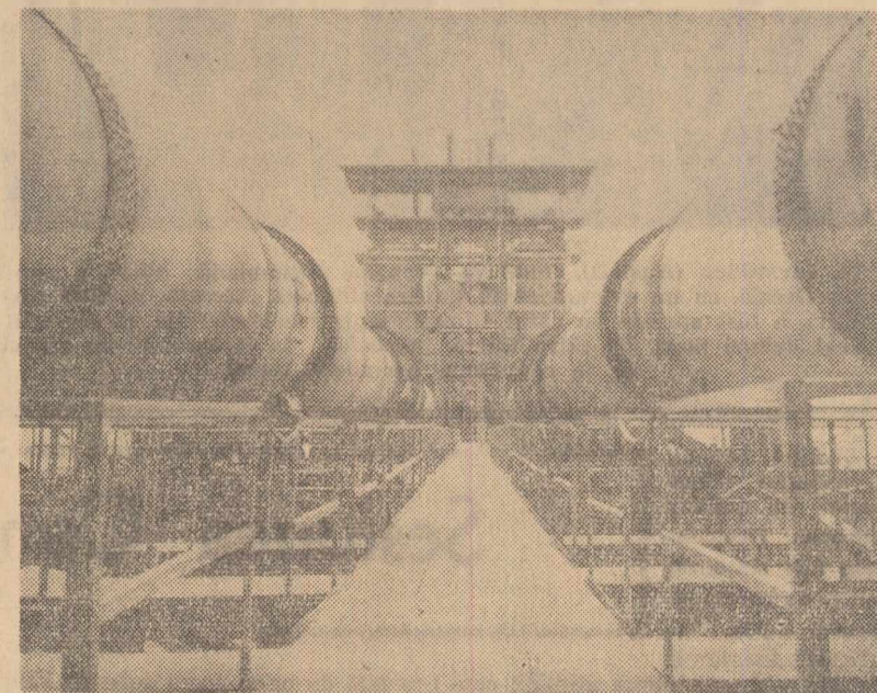
Cuptoarele rotative ale fabricii de acid sulfuric de la Wizow (R. P. Polonă)
