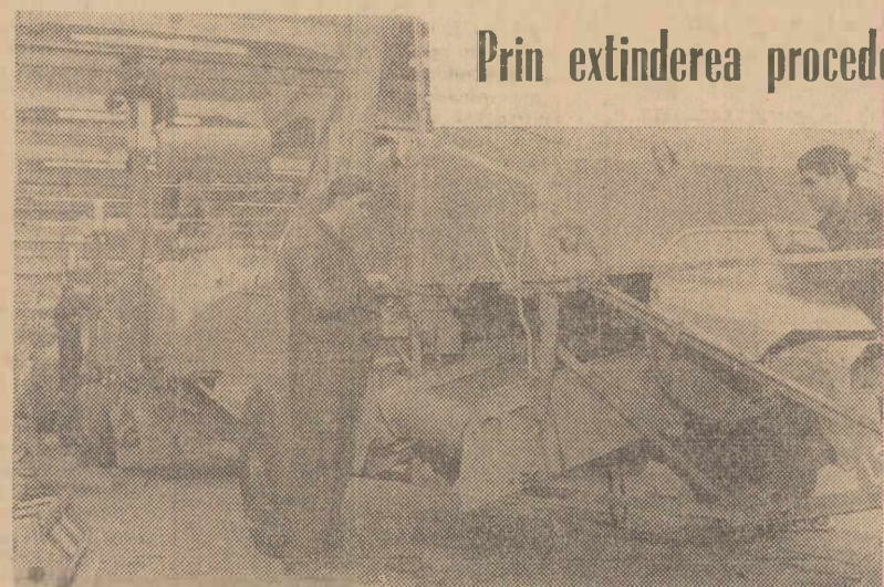
Uzina de mașini agricole „Semănătoarea”. Se montează un nou lot de combine. Foto: I. AGERPRES
