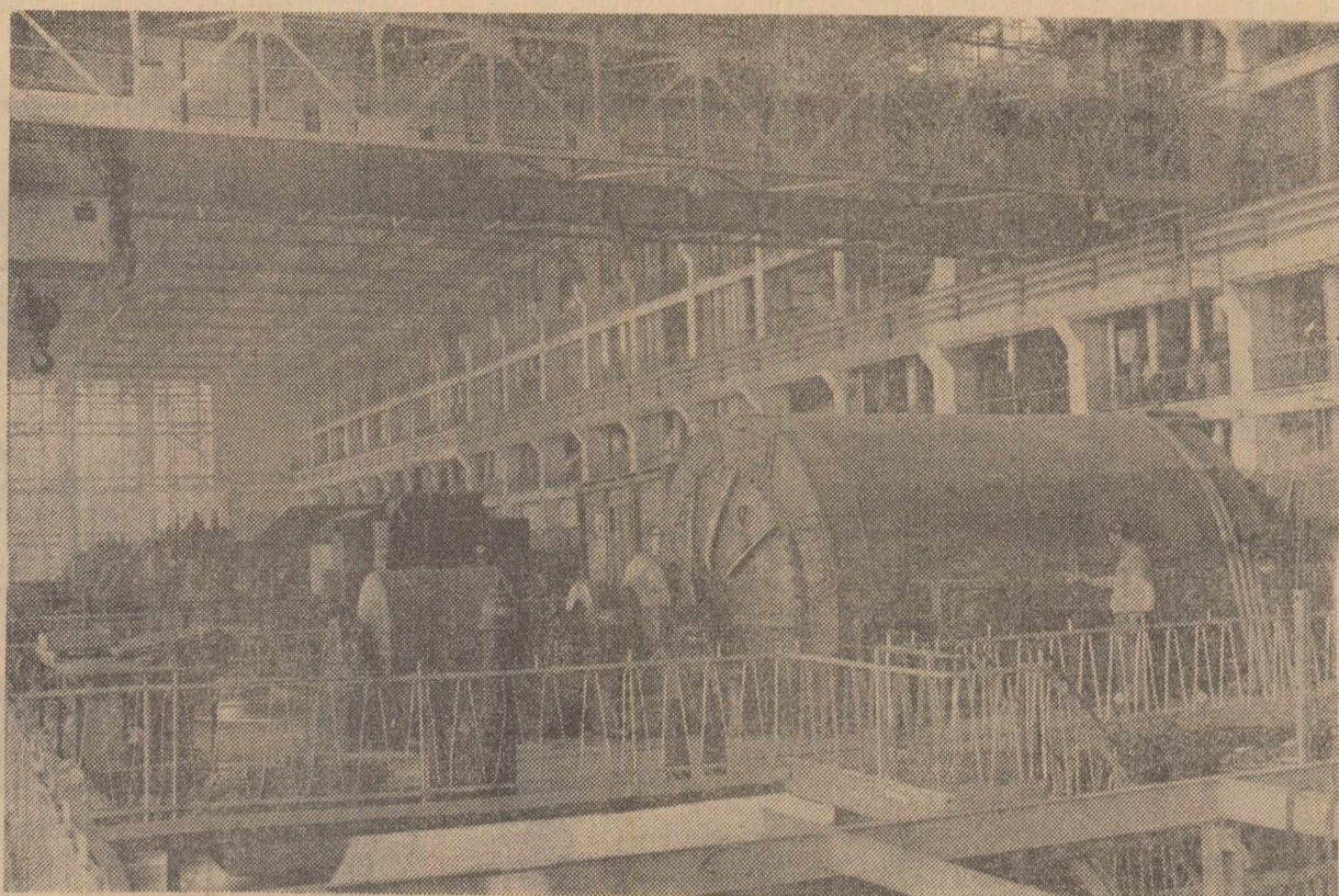
Recent a intrat în funcțiune la Termocentrala de la Brazi grupul turbo-generator nr. 4. În clișeu: Noul agregat. Foto: I. AGERPRES
