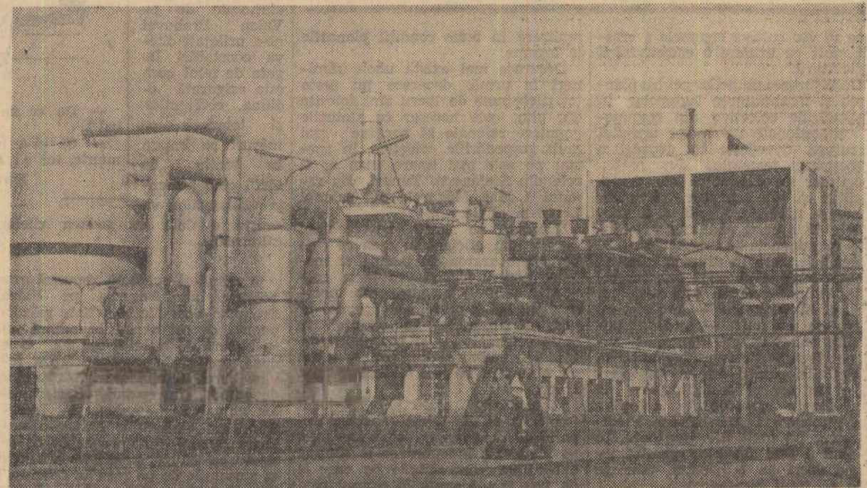
Uzinele de acid sulfuric și superfosfat din Năvodari au produs în primul trimestru al anului aproape 70.000 tone îngrășăminte chimice simple și granulate. În elușu: Noua linie de acid sulfuric a uzinei, dată anul trecut în funcțiune.
