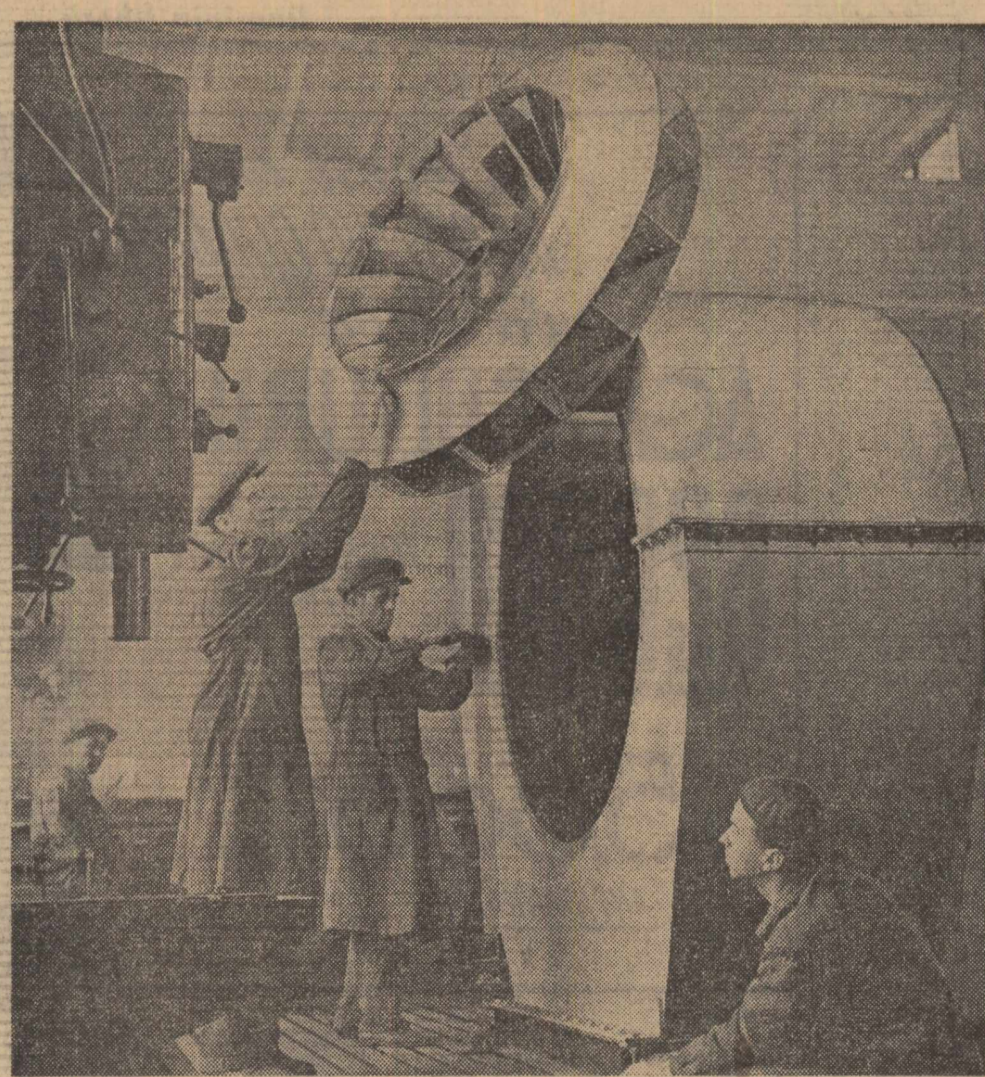
Colectivul întreprinderii metalurgice „Dealul Spirii” din Capitală produce diferite tipuri de mașini de stropit și prăfuit, necesare combaterii bolilor și dăunătorilor în agricultură. De asemenea, aici se produc și ventilatoare industriale. În clișeu: Șeful brigăzii de montaj ventilatoare Tudor Dobre, împreună cu lucrătorii Petre Gheorghe și Cristache Barbu pregătesc montarea rotorului la un ventilator.
