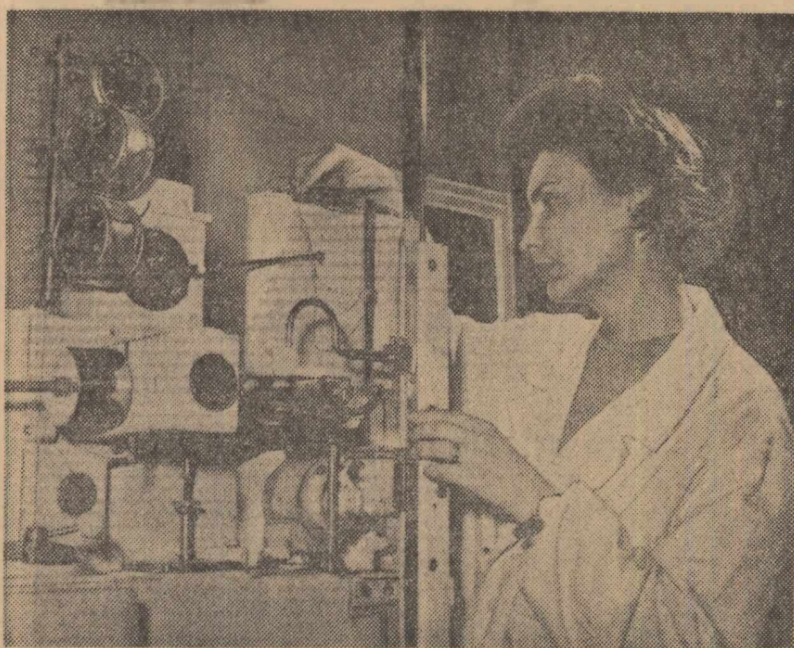
Laboratorul de studii al calității grîului din cadrul Institutului de cercetări agricole, desfășoară o rodnică activitate. În clișeu: inginerul chimist Lidia Cernescu, urmărind la extensograf rezistența aluatului dintr-un nou soi de grîu creat în țara noastră
