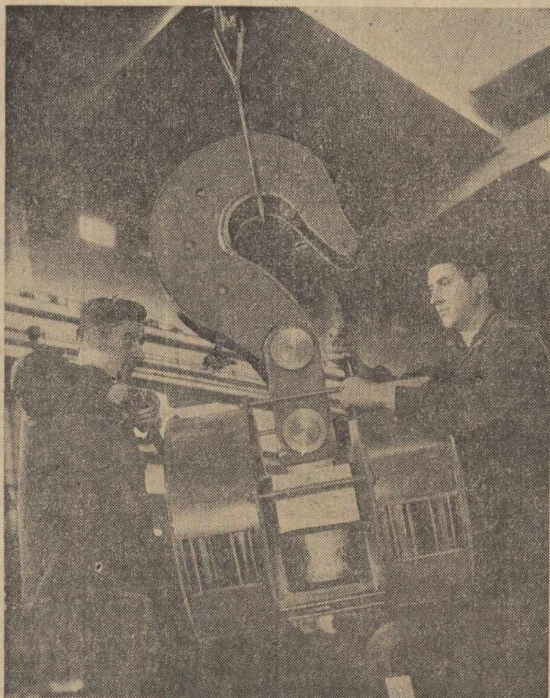
Brigada de lăcătuși de la Uzinele metalurgice din Timișoara își depășește cu regularitate sarcinile de plan, făcând în același timp lucrări de bună calitate. În clipă: lăcătușii Ion Farcas și Ștefan Orlu, doi din fruntașii brigăzii, lucrând la asamblarea cilindrilor pentru macaraua de 30 tone. Foto: AGERPRES
