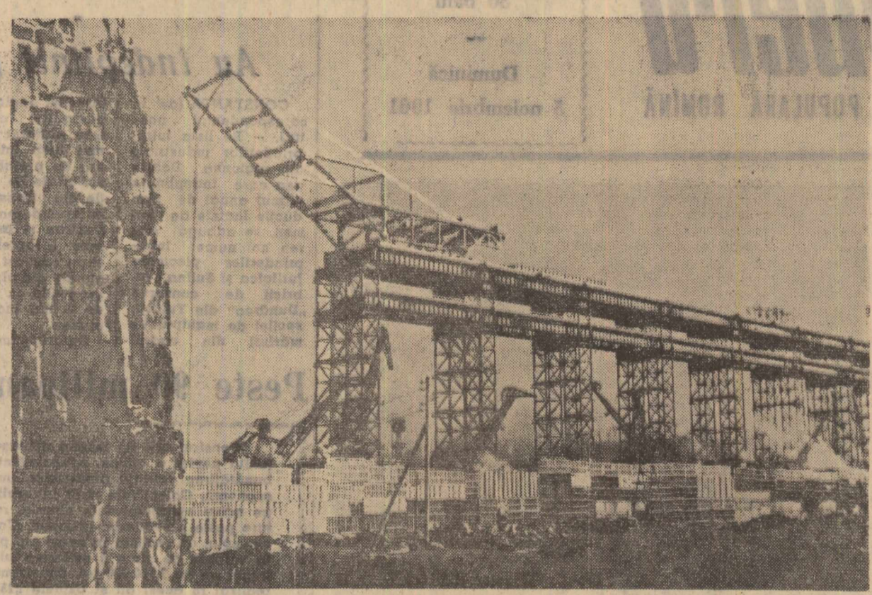
De curînd, la hidrocentrale de la Bratsk, de pe fluviul Angara (Siberia răsăriteană), a fost montat primul turbogenerator, a cărui înălțime este cît a unei clădiri cu patru etaje, iar puterea lui este de 225.000 kW. Pe barajul hidrocentral de la Bratsk, vor fi instalate 20 de turbogeneratoare de acest fel. Construcțiile acestui gigant energetic (cel mai mare din lume) tînesc prin dimensiunile lor: înălțimea barajului trece de 100 metri, iar capacitatea lacului de acumulare va fi de aproximativ 180 miliarde metri cubi de apă. În clișeu: Estacada pentru transportarea betonului pe șantierul hidrocentral de la Bratsk.
