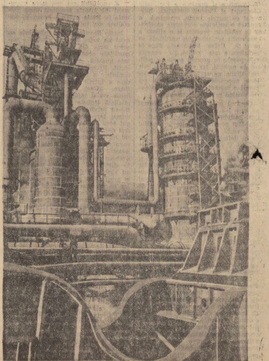
La uzina metalurgică din Vorosilovsk, regiunea Lugan, s-a reconstruit un furnal după o metodă cu totul originală. Pe un stand special, pe role, la 20 m. depărtare de vechiul furnal, a început montarea celui nou. Cînd înălțimea noului furnal a ajuns la 70 m și la o greutate de peste 3000 tone, el a fost deplasat — cu ajutorul unor cricuri — macarale — pe fundația vechiului furnal. În clișeu: Furnalul reconstruit.
