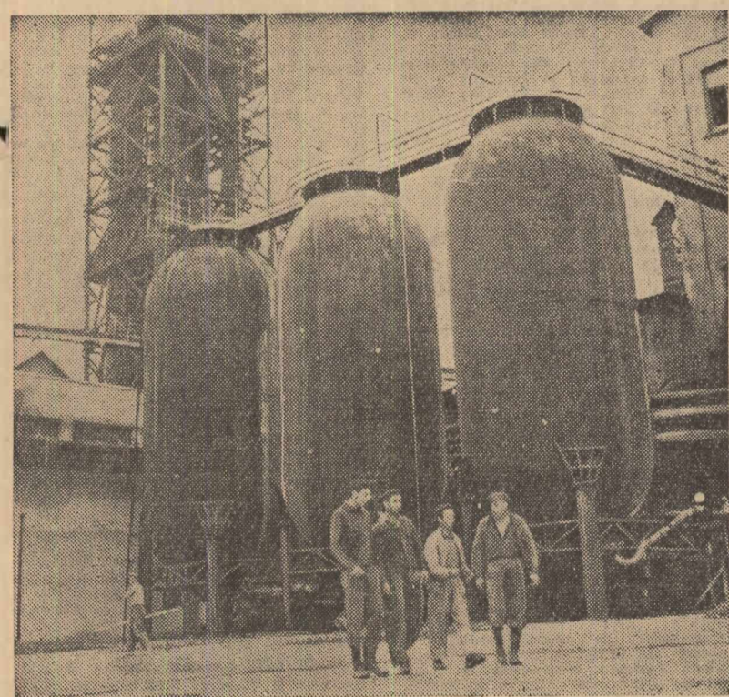
Instalația de prelucrare și concentrare a soluțiilor de fierbere dețin în funcțiune anul acesta la fabrica „Steaua roșie” din Bacău
