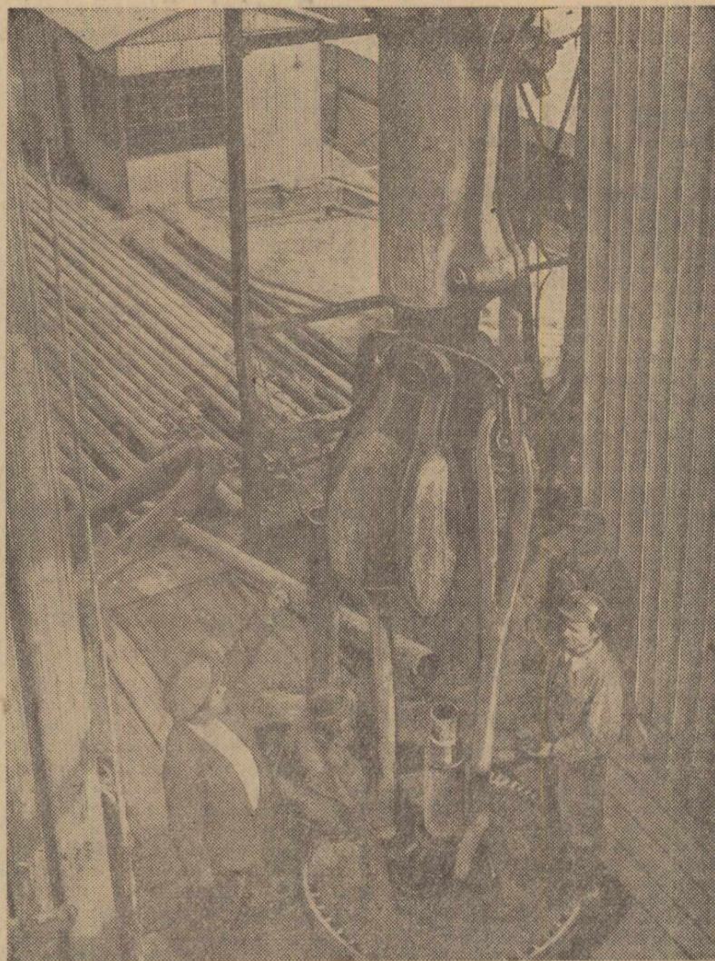
La sonda nr. 502 de la schela Boldești s-a introdus pentru prima oară în țară electrobrurul. Cu ajutorul acestor moderne instalații sovietice s-au realizat viteze medii de foraj de patru ori mai mari decât cu masa rotativă. Brigăzile conduse de comunistul Gheorghe Aurel, care se numără printre cele frunțose din schela Boldești, l-au revenit clăstea de a foră această primă sondă cu electrobrurul. În clișeu: Maistrul Gheorghe Aurel dînd îndrumări tehnice unor membri din brigadă. Foto: AGERPRES
