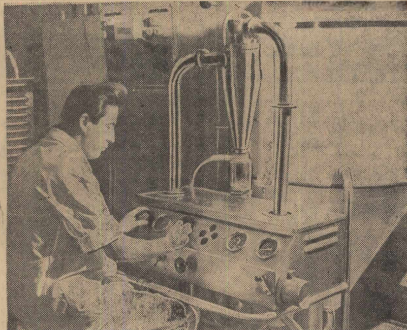
La Institutul de cercetări alimentare din București se rezolvă probleme științifice legate direct de desigurarea proceselor de producție în sectoarele industriale. În clădire: tehnicianul Constantin Ciupercă urmărește, cu ajutorul liniei experimentale, procesul de uscarea a lăptelui praf dietetic la aparatul de pulverizare
