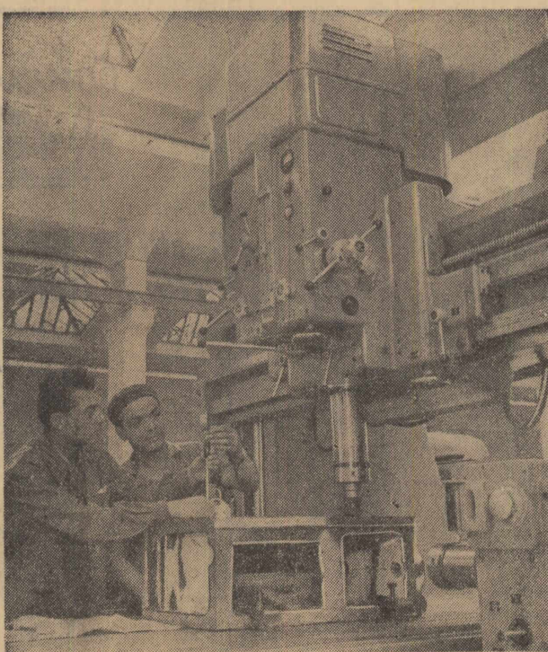
În cadrul uzinelor „23 August” din Capitală a fost de curînd amenajată o secție de sculărie dotată cu mașini moderne. În clădire: Inginerul Ion Burlacu, șeful secției sculărie și Constantin Ficu controlează execuția unei plesse
