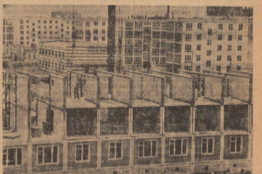
Cliseul de mai sus reprezintă un aspect de pe șantierul din partea de nord-vest a Moscovei, unde se ridică 27 blocuri din panouri mari prefabricate, pe o suprafață de peste 50.000 m.p.
