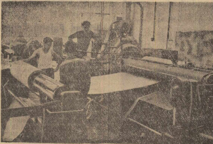
La fabrica de placaje — prima unitate, dată în funcțiune — mașina de derulare transformă buștenii în foi subțiri de furnir.
