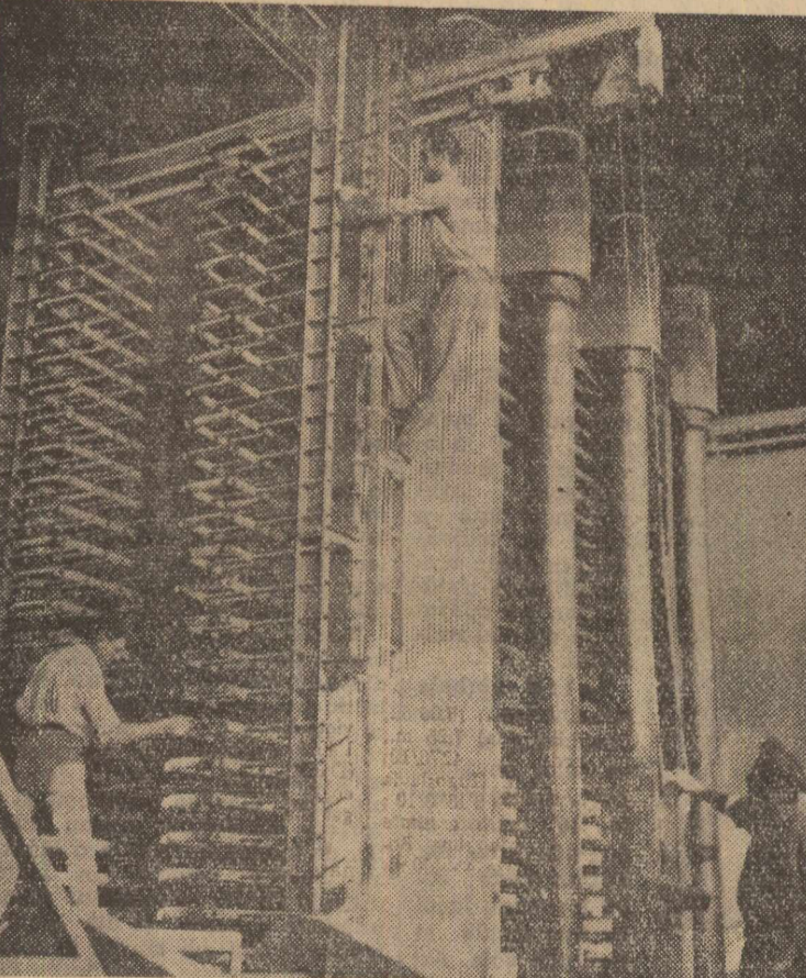
Uruga presă a fabricii de plăci fibro-lemnoase a fost montată. Fotografia: NICU VASILE
