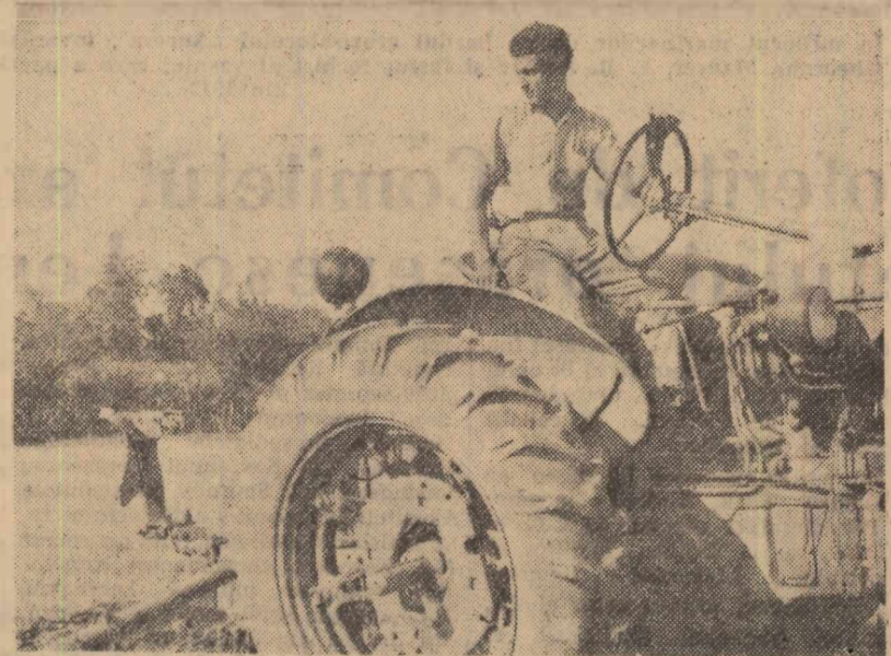
La gospodăria colectivă din Ciupercent, regiunea București, se acordă o atenție deosebită executării arăturii adînci de vară pe suprafețe cât mai mari. În clișeu: tractoriul Vașle Done de la S.M.T. Traian, în timpul lucrului. Foto: N. SCARLET
