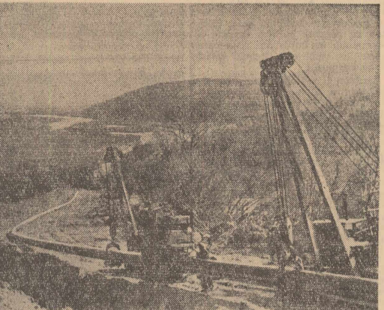
În clișeu: Lucrările de montare a conductei internaționale de petrol „Drujba” în regiunea Lvov. Curățirea și izolarea conductelor pe care îl traseu accidentat care cuprinde o întindere de peste 100 km.
