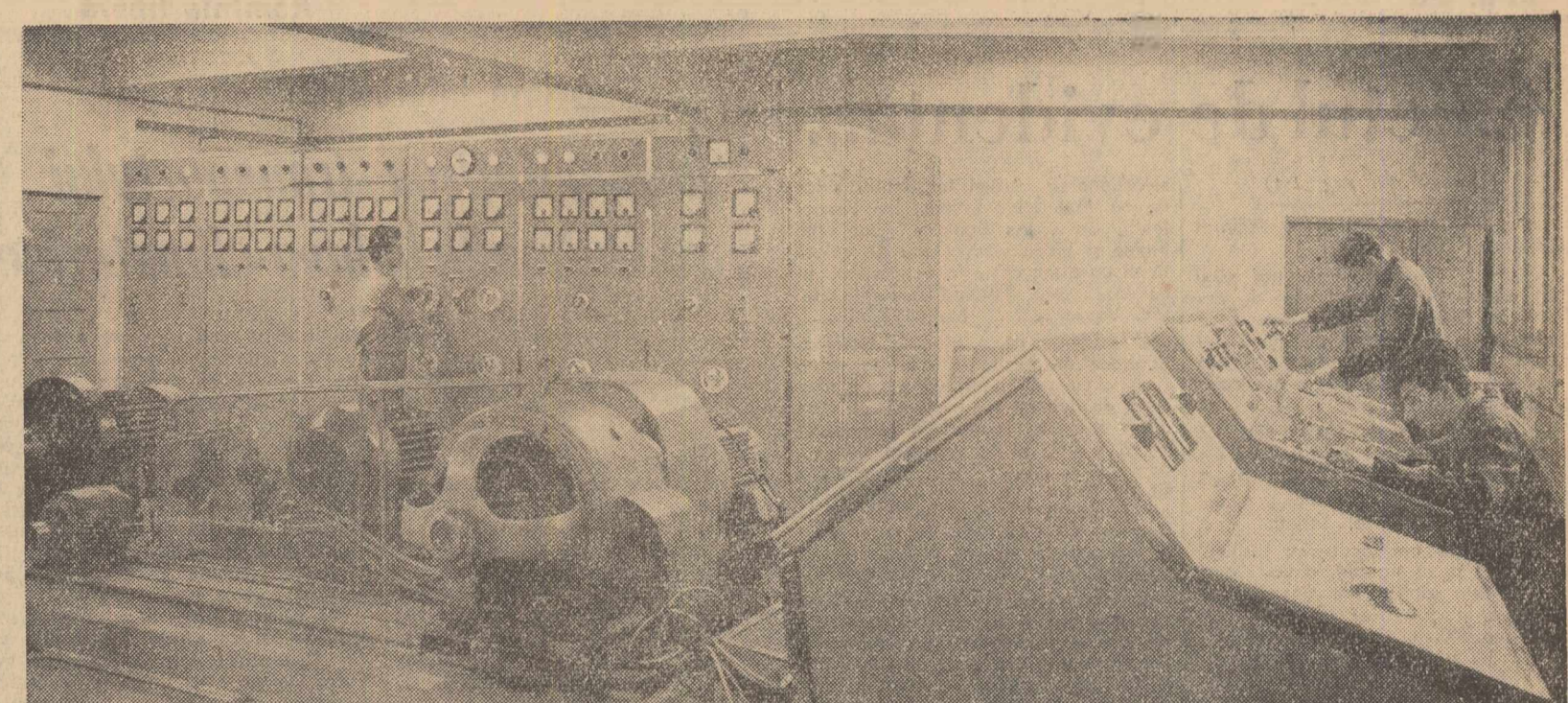
Colectivul de muncă de la întreprinderea „Electromotor” Timișoara, are în atenție permanentă modernizarea a produselor uzinei. La începutul acestui an a fost dat aici în funcțiune un stand de încercări-tip al motoarelor. Această instalație reduce timpul de încercare al motoarelor electrice cu 50 la sută față de cea veche. În clișeu: standul de încercări al motoarelor Foto: A. CONSTANTINESCU
