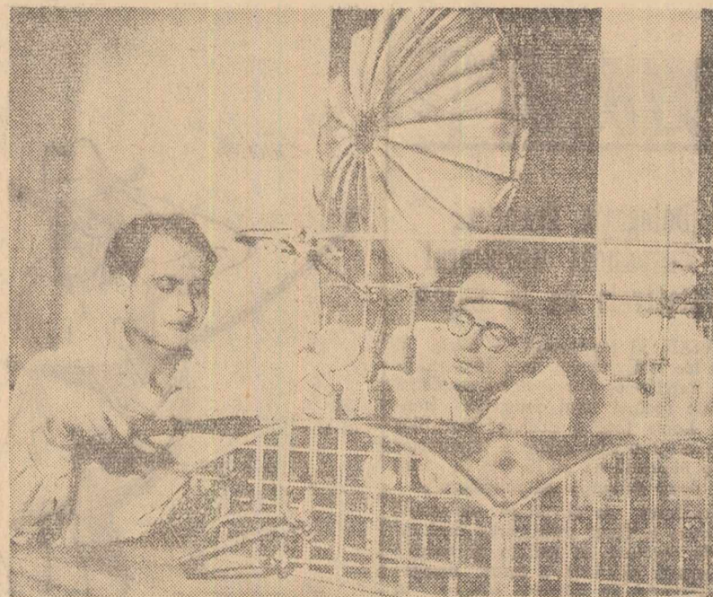
În laboratorul de studii pe modele al Institutului de cercetări în construcții și economia construcțiilor, ing. E. Nicolau și tehnicianul I. Ispas execută un studiu al comportării de ansamblu al unei construcții cu ajutorul modelelor la scară redusă.
