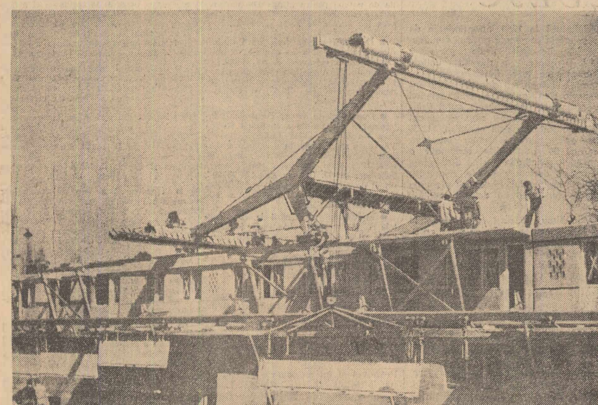
Pe șantierul nr. 2 Grivița Rosie și-a făcut apariția de curînd o nouă macara. Este vorba de macaraua reversibilă, un sprijin prețios pentru constructorii deoarece noul produs prezintă multe avantaje ușurînd mult munca constructorilor, contribuînd în același timp la accelerarea lucrărilor de montare a prefabricatelor din beton. În clișeu: Macaraua reversibilă pe șantier. Foto: MIHAI POPESCU
