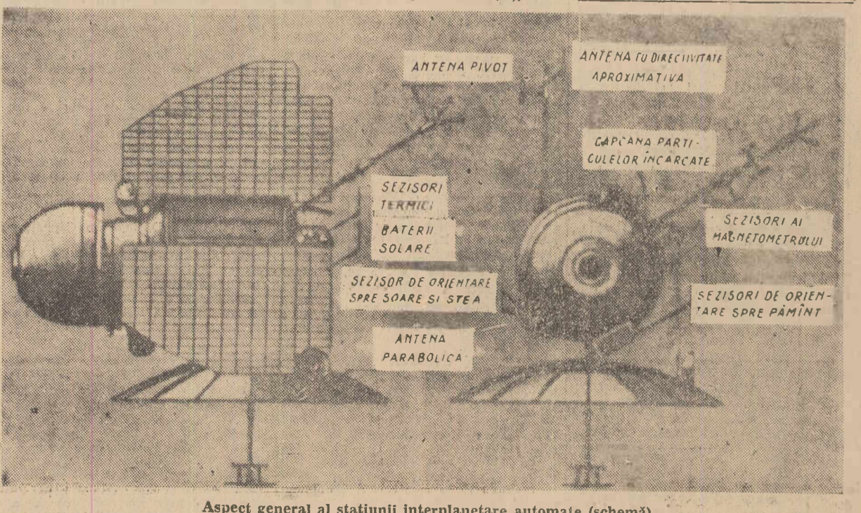
Aspect general al stațiunii interplanetare automate (schemă).
