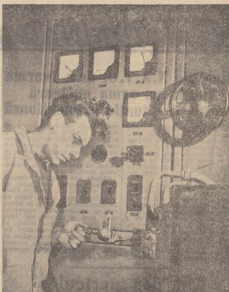
La uzinele de tractoare „Ernst Thälmann” din Brașov, secția de tratamente termice a fost reorganizată și modernizată pentru a face mai bine față necesităților producției de tractoare în plină creștere. În clipă: Un aspect din sectorul de călărie cu curent de înaltă frecvență. Ernst Gune lucrează la noul generator electric, executînd călărea parțială a furcii cutiei de viteză.
