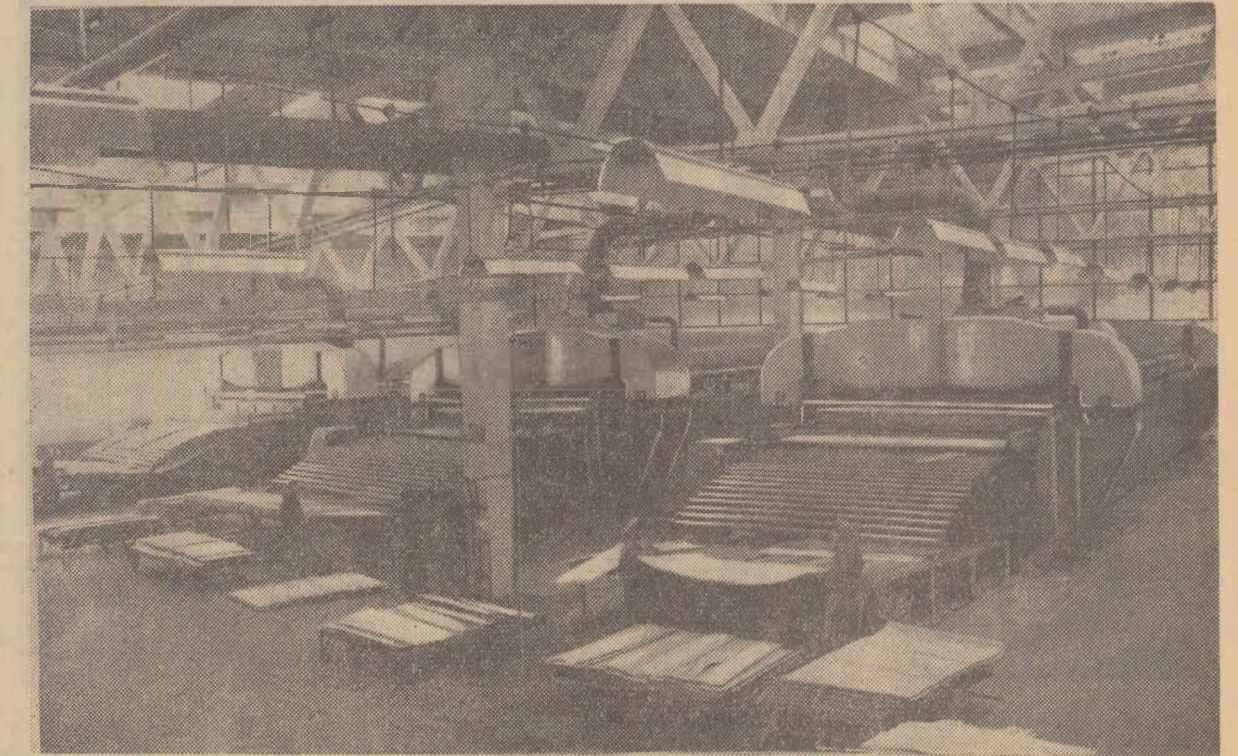
Un aspect de la uscătoarele de furnire a fabricii de placaje.
