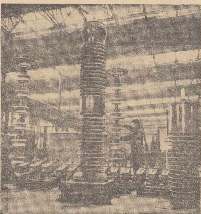
La standul de control tehnic pentru aparatul electric de înaltă tensiune din cadrul uzinelor „Electroputere”-Craiova se pregătesc pentru verificare întreprinderile în ulei puțin (I.U.P.) de 15 Kv. 600 A. Foto: (AGERPRES)
