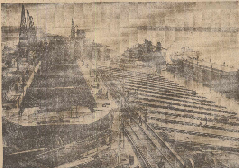
Vederea panoramică a șantierului naval de la Oltenița. Pe cale, mai multe vase în construcție.
