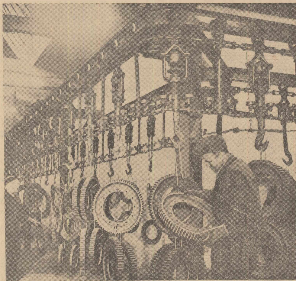
Rînd pe rînd, transportorul scoate piesele gata sablate din tunelul automat. (Clicseul de sus). Ultima fază din procesul tehnologic. Tractoarele au ajuns pe banda de montaj (Clicseul de jos).
