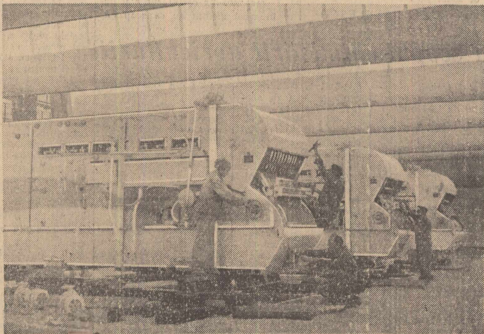
Cliseul din stînga: La secția spălat sticle se montează mașinile. Cliseul din dreapta: În sala de mașini frigorifice compresoarele au fost montate. În prezent se face rodajul.
