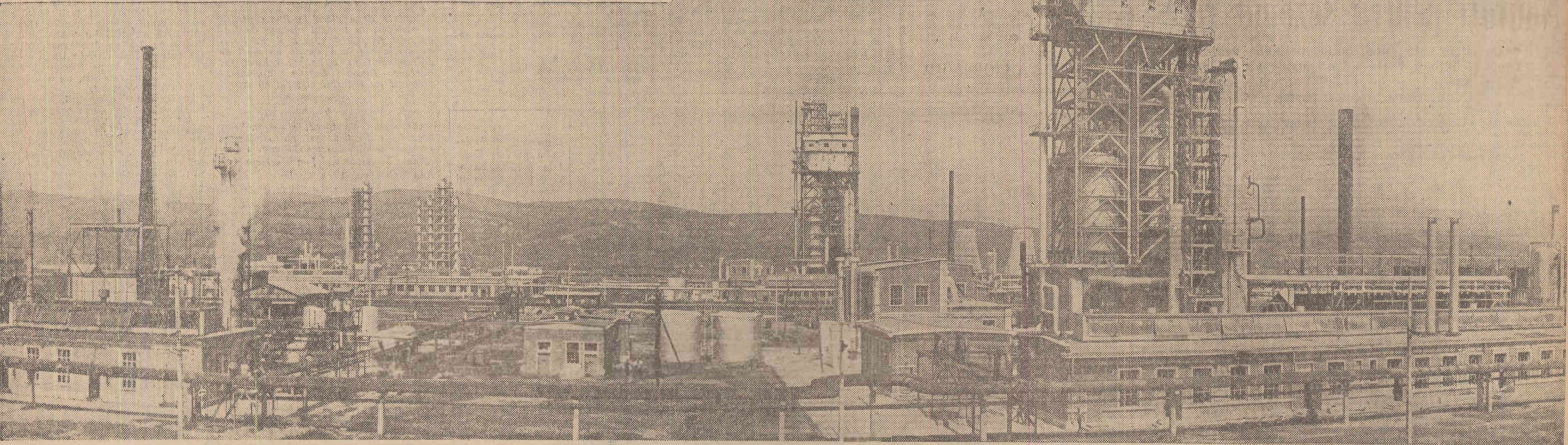
Vedere generală a rafinăriei din Onești. În prim plan: Instalația de cracare catalitică nr. 2 intrată în funcțiune în cinstea zilei de 23 August.
