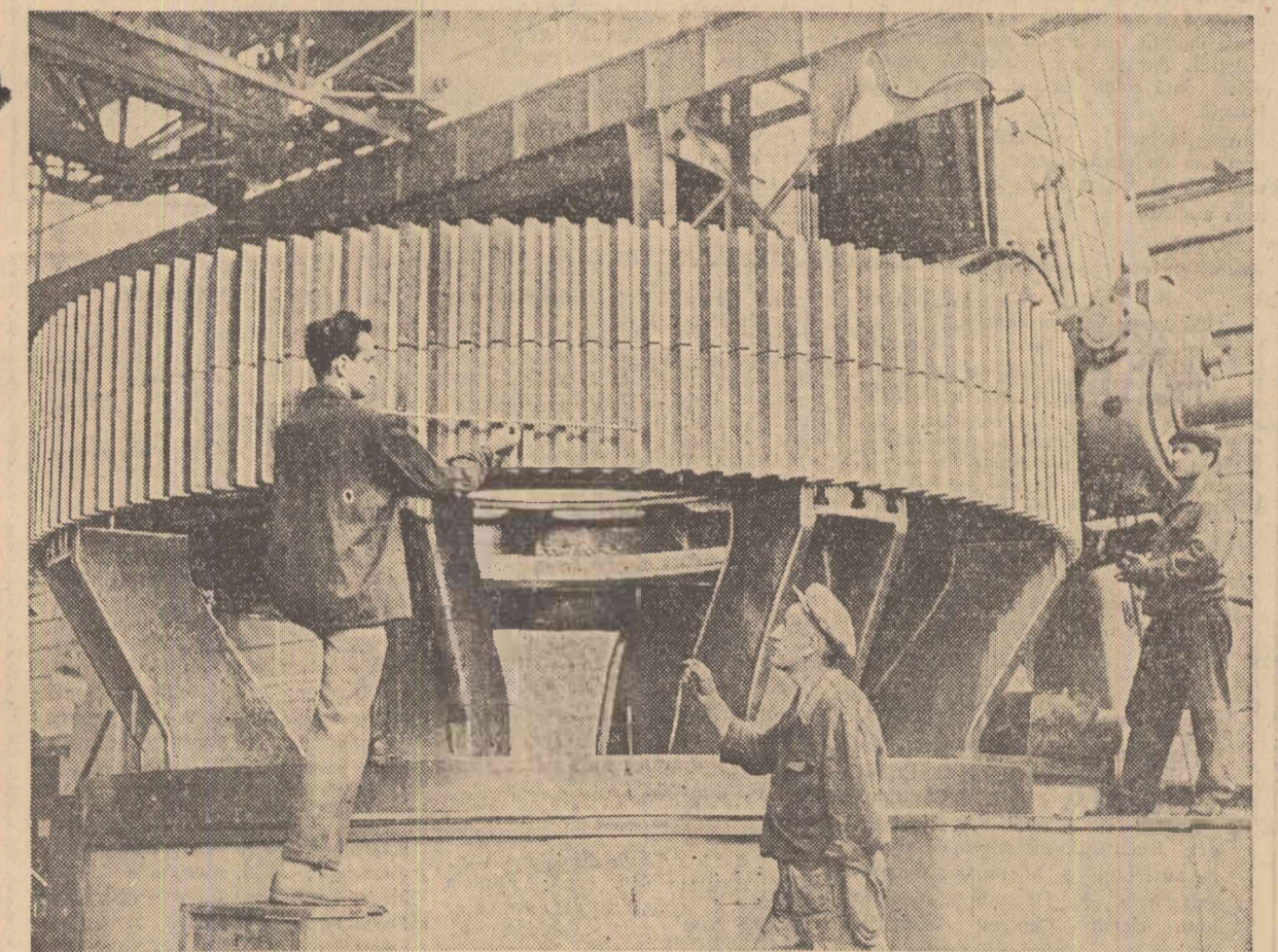
La atelierul de mecanică grea de la Uzinele „23 August” din Capitală lucrează, printre alii frunțași, inginerul Marin Stancu, strungarul Ștefan Munteanu și lăcătușul monitor Gh. Bungeanu. Iată-l în clăusel nostru verificînd cota peste dinți a celor două roți care vor pleca peste puțină vreme la morile de ciment. Fiecare din aceste roți are un diametru de circa 4300 mm și o greutate de 13 tone.
