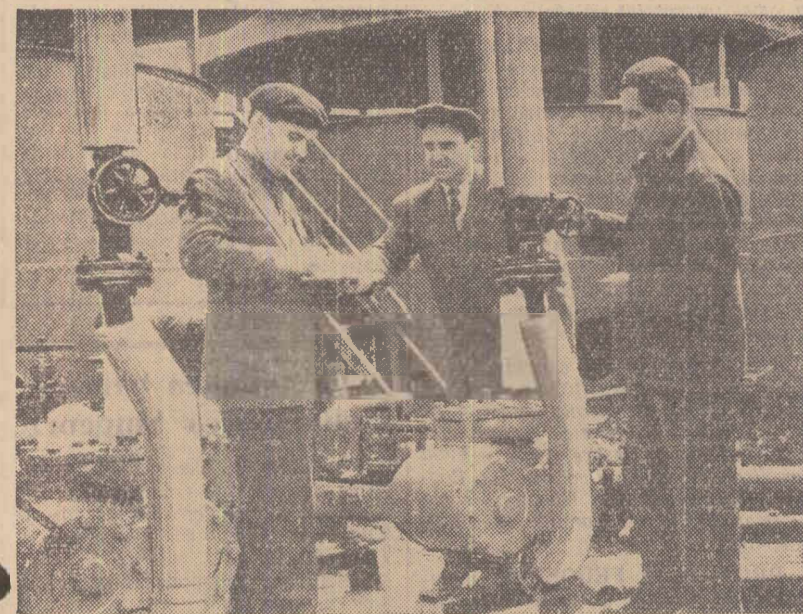
Ing. Gheorghe Pescaru, plumbitorul Petre I. Nicolae și responsabilul cabinetului tehnic, tovarășul Ion Nicolae, discută despre felul cum vor fi dirijate cu ajutorul pompei speciale gudroanele acide în instalație.
