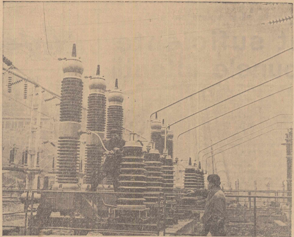
La hidrocentrala „V. I. Lenin” de la Stejaru (Bicaz), concomitent cu montarea turbinelor se montează și stațiile de transformare. În clădire: Lăcătușul stației, Gh. Bogde și sudorul Petre Fermeșanu, montează ultimele legături ale circuitelor primare ale întrerupătoarelor cu aer comprimat la una din stațiile de transformare de 110 kW. Foto: NICU VASILB
