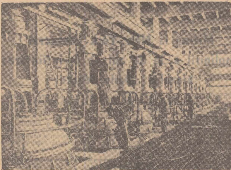
Pe șantierul Combinatului de cauciuc sintetic de la Onești, lucrările de construcție și montaj avansează pe zi ce trece. În clădire: muncitorii lucrează la instalarea amestecătoarelor în hala secției de polimerizare.
