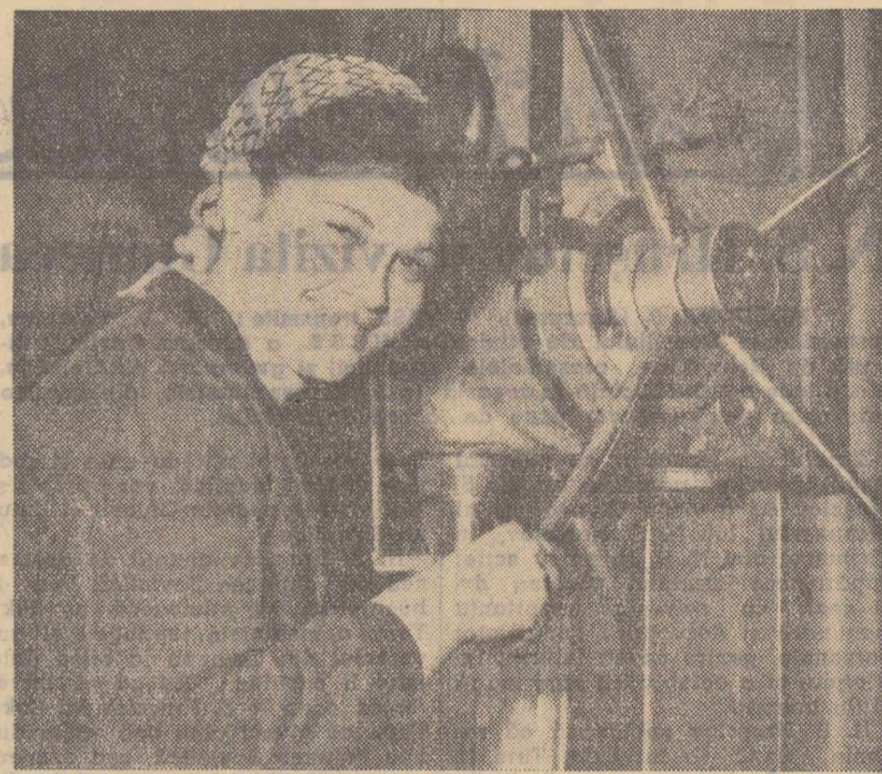
Utemista Geta Enache, muncitoare la fabrica de rulmenți din Birlad, lucrează în atelierul de frezat colivii pentru rulmenți. Folosind rațional cele 480 de minute și capacitatea de lucru a mașinii, ea își depășește zilnic sarcinile de plan cu 20—25 la sută. De multă vreme ea se situează printre tinerii fruntași din secția în care lucrează.
