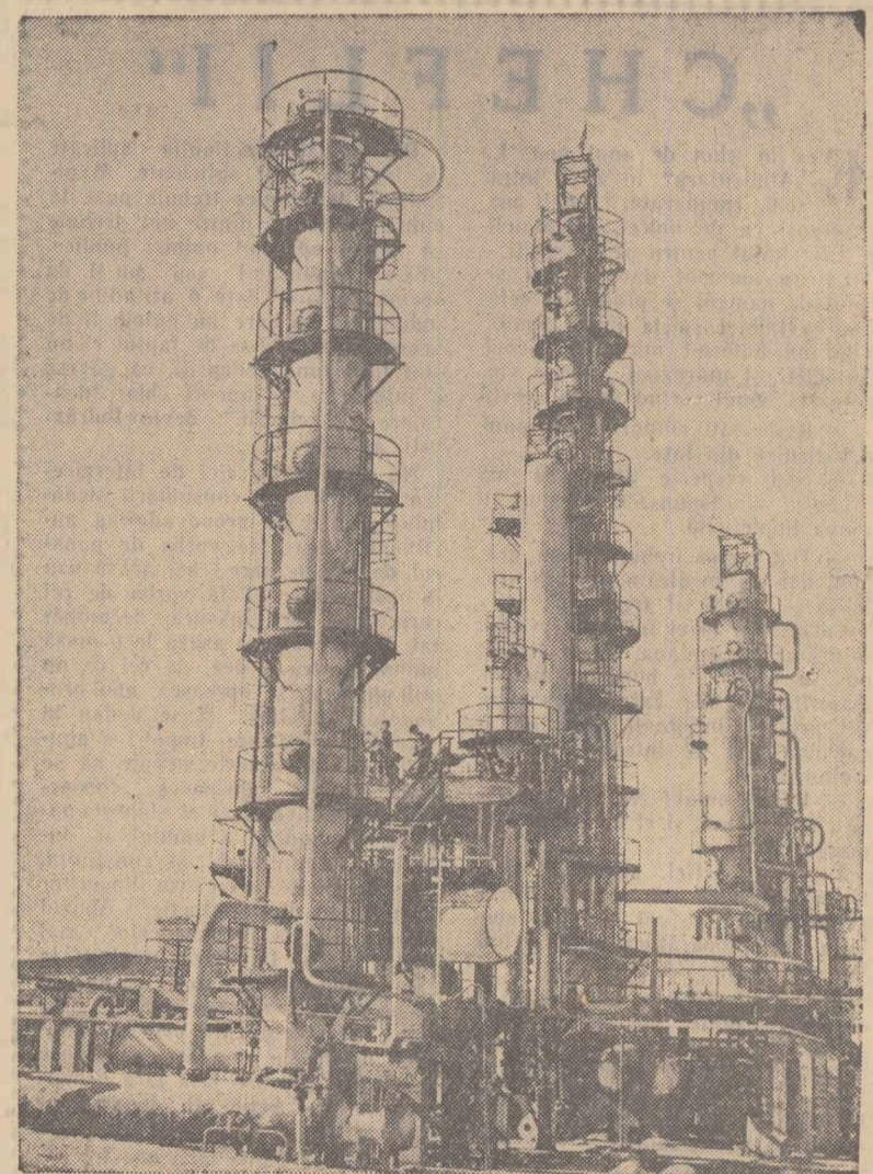
Cea de a doua parte a construcțiilor din cadrul rafinării de petrol de la Tușantzu a fost terminată înainte de termen. În prezent funcționează instalația de distilare, secția de cracare termică și termocentrala. Prin terminarea noilor secții sporște cantitatea de produse petroliere dobîndită din tîțeiul bazinului petrolier Karamai. În fotografie: Aspect de pe teritoriul rafinării de petrol de la Tușantzu
