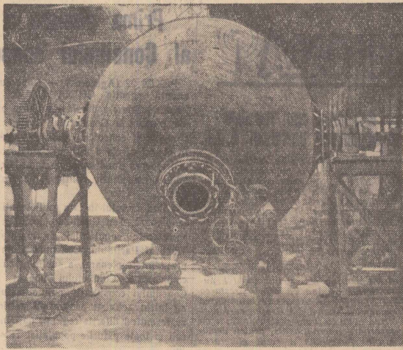
Printre produsele noi realizate în acest an de colectivul uzinelor metalurgice „Progresul” din Brăila se numără și autoclava sferică pentru prepararea furfurului. În elisaur. Autoclava sferică care se face ultima revizuire înainte de expediere.
