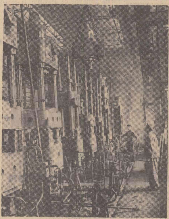
Montarea unei prese de 200 tone la uzina de prese hidro-draulice din Orenburg (U.R.S.S.)
