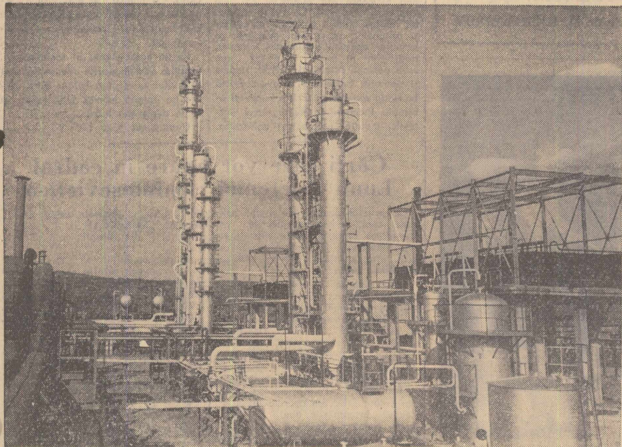
Instalația de absorbție și fracționarea gazelor de la Rafinaria nr. 10 Onești.
